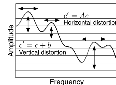
図2 ベクトル b および行列 A によるスペクトル変形 Fig.2 Two kinds of spectral distortions caused by vector b and matrix A .
