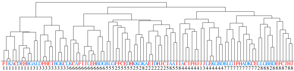
図 3: 構造的表象に基づく英語発音分類
