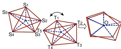
図 4: 回転とシフトによる構造群の接近と構造間距離
