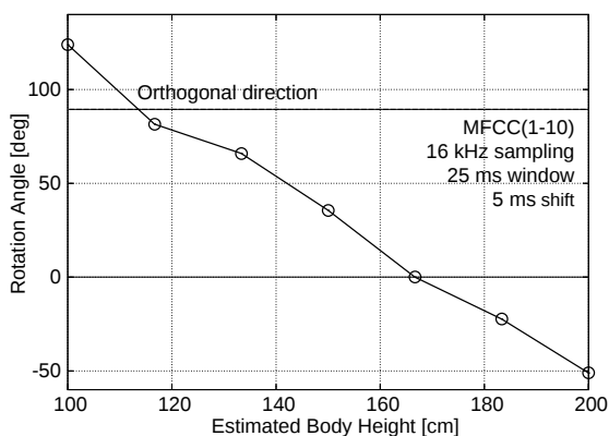
図 10 音色の動的変化パターンの方成分が示す身長依存性
