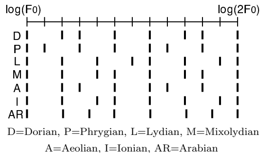
図2 6種類の古典的教会音階とアラビア音階
