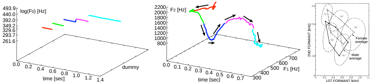
図3 F_0 の動的変化としての CDEFG と音色の動的変化としての /aiueo/, 及び、日本語母音図
