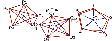
図8 回転及び平行移動を行なう音響照合
