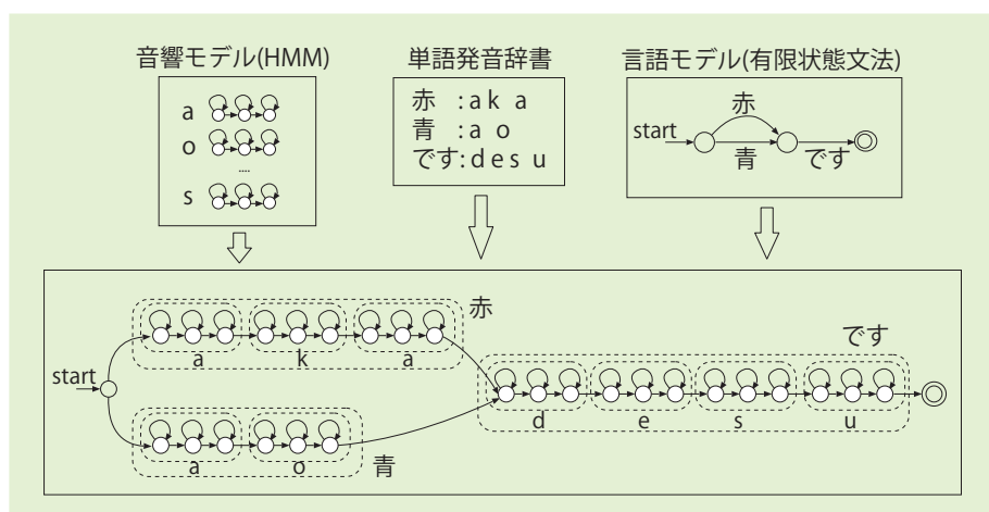
図-1 音声認識における探索空間表現
