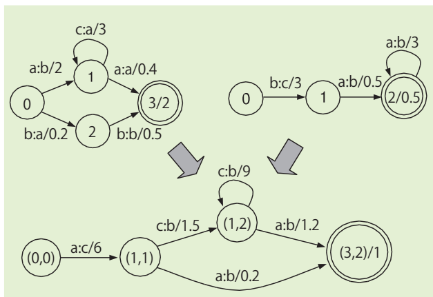
図-8 WFSTの合成 (composition)
