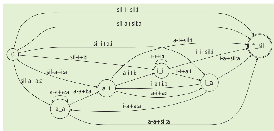
図-10 トライフォン接続制約を表す WFS
