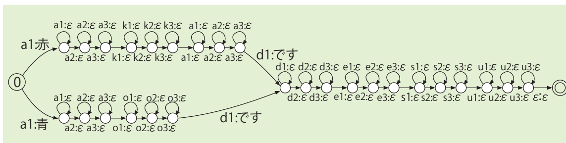
図-9 WFSTによる探索空間表現
