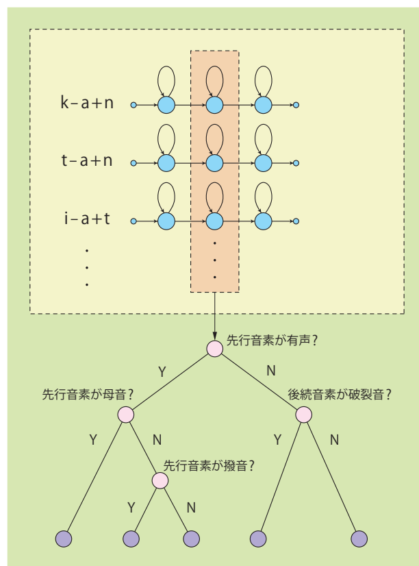
図-4 HMMのコンテキストクラスタリング
