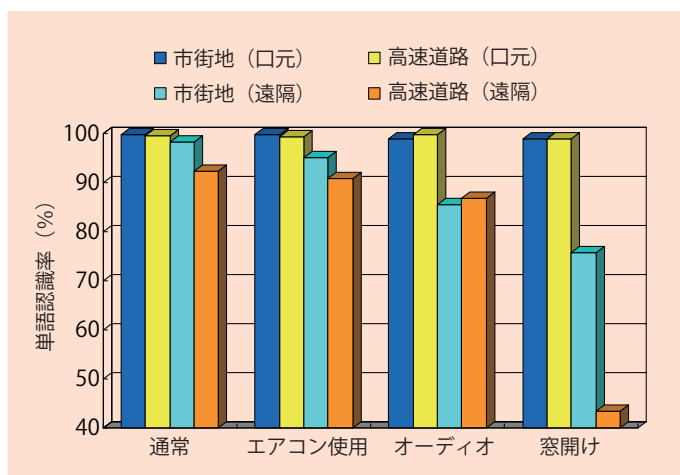
図-1 小語彙の単語発声に対する車内音声認識性能
