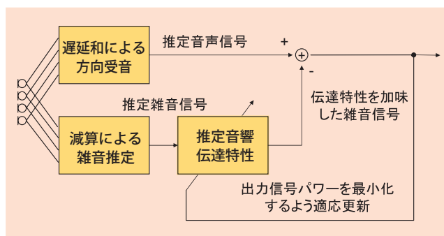
図-5 適応的マイクロホンアレー (Griffith-Jim 型ビームフォーマ) の構成
