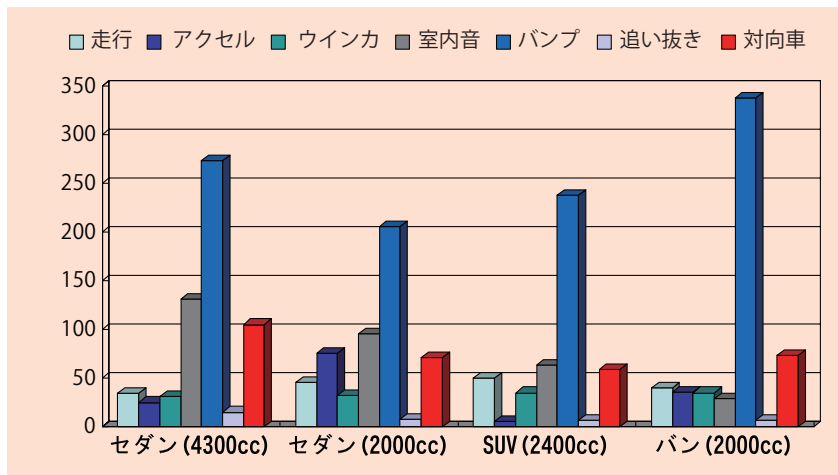
図-3 定常走行中の自動車内の雑音イベント（1時間に聞き取れた回数）
