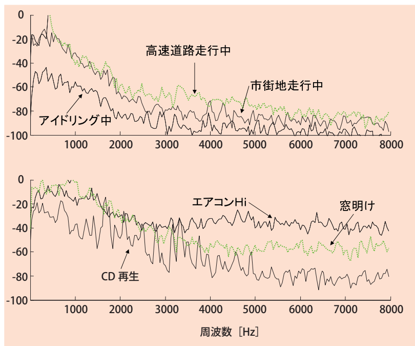
図-4 車内雑音の平均スペクトル
