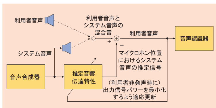
図-6 バージインを実現するための案内音声の消去
