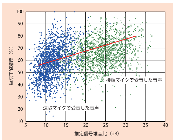
図-2 SN比のばらつきと大語彙連続音声認識に対する車内音声認識性能
