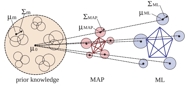
図 4 音声事象分布の最大事後確率推定
