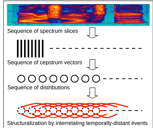
図 2 一発声の構造化
