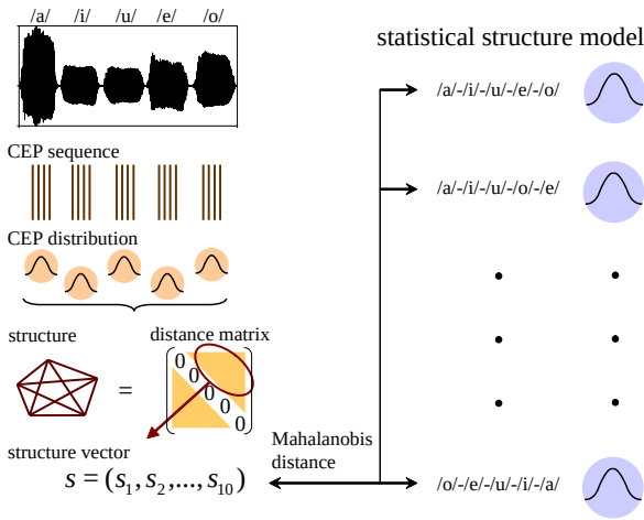
図5 構造を用いた日本語母音系列の自動認識
